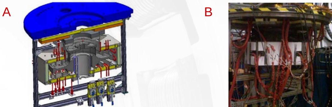
Figure-9 – Thermal Gradient Test Rig. A) CAD model and B) Actual thermal gradient oven.
